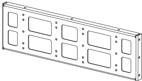
(1) 3U DIN Rail Back Panel
